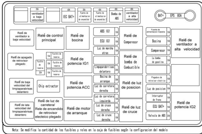
Caja de fusibles del compartimento del motor
